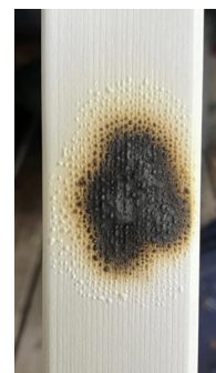
Couche protectrice (meringue) formée sur un Profil Quadri 40 x 40
